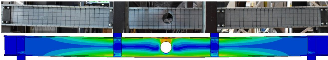
(d) W240-L4-UH1
