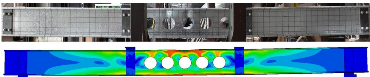
(l) W290-L4-UH5
