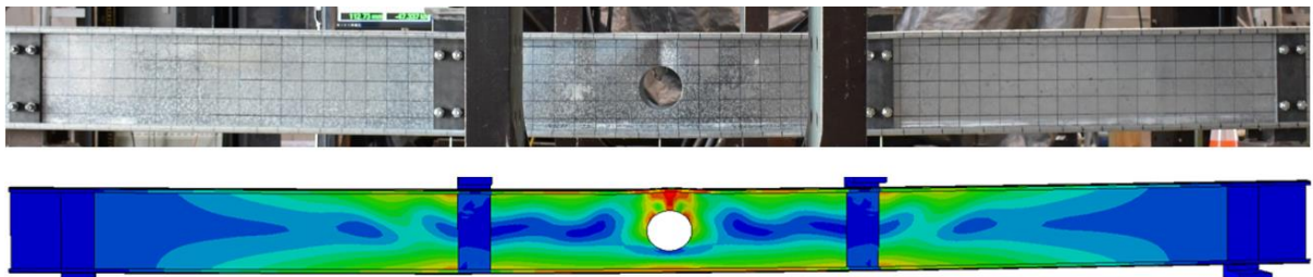
(j) W290-L4-UH1
